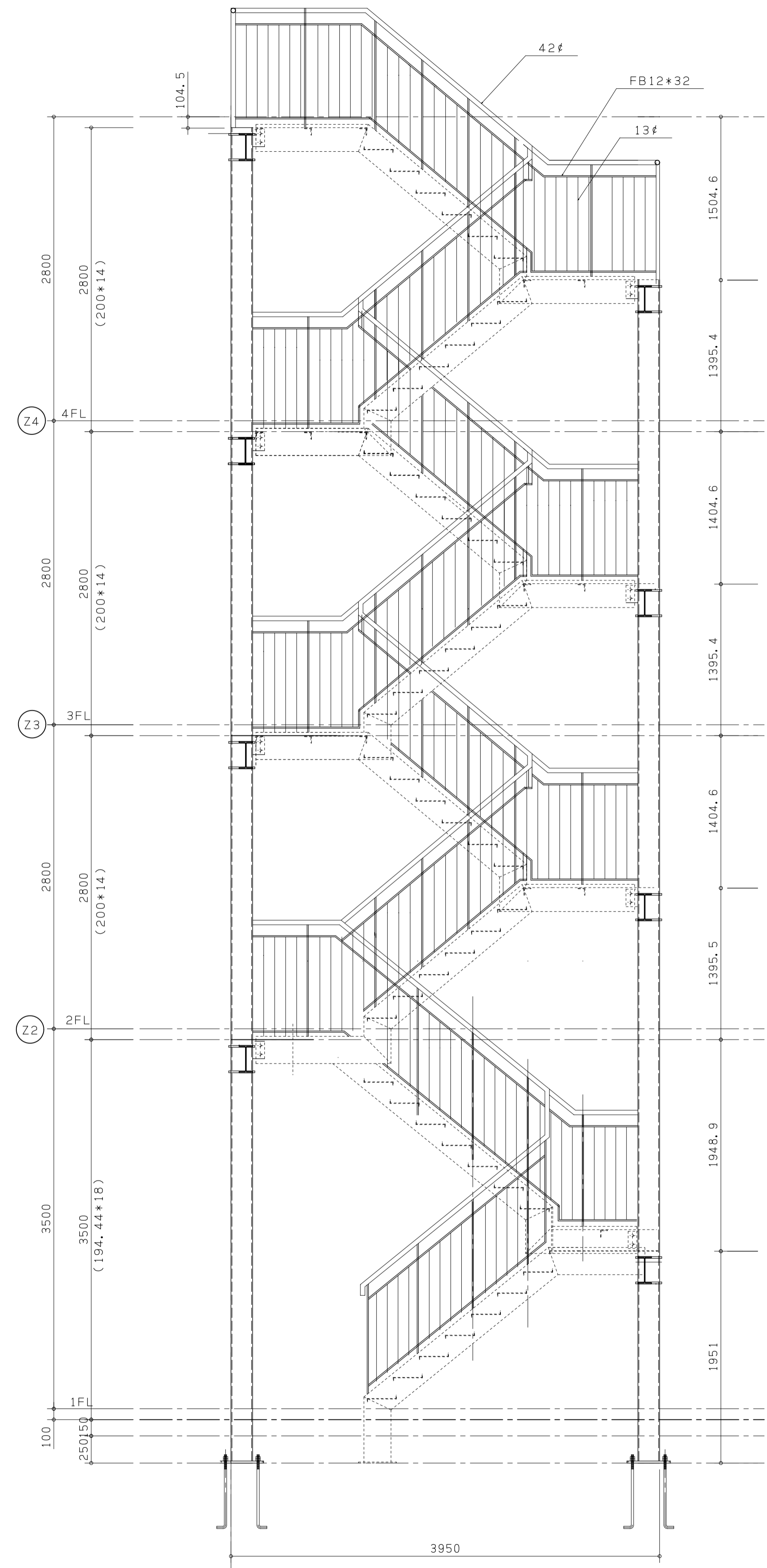
A---A 断面図 S=1:30
