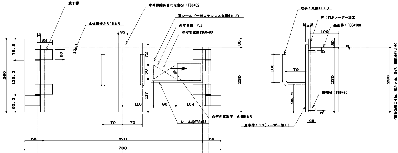
正面図 S=1:4
