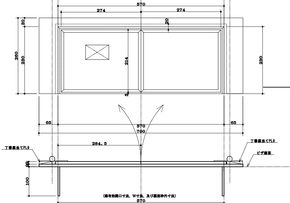
正面図 S=1:4
