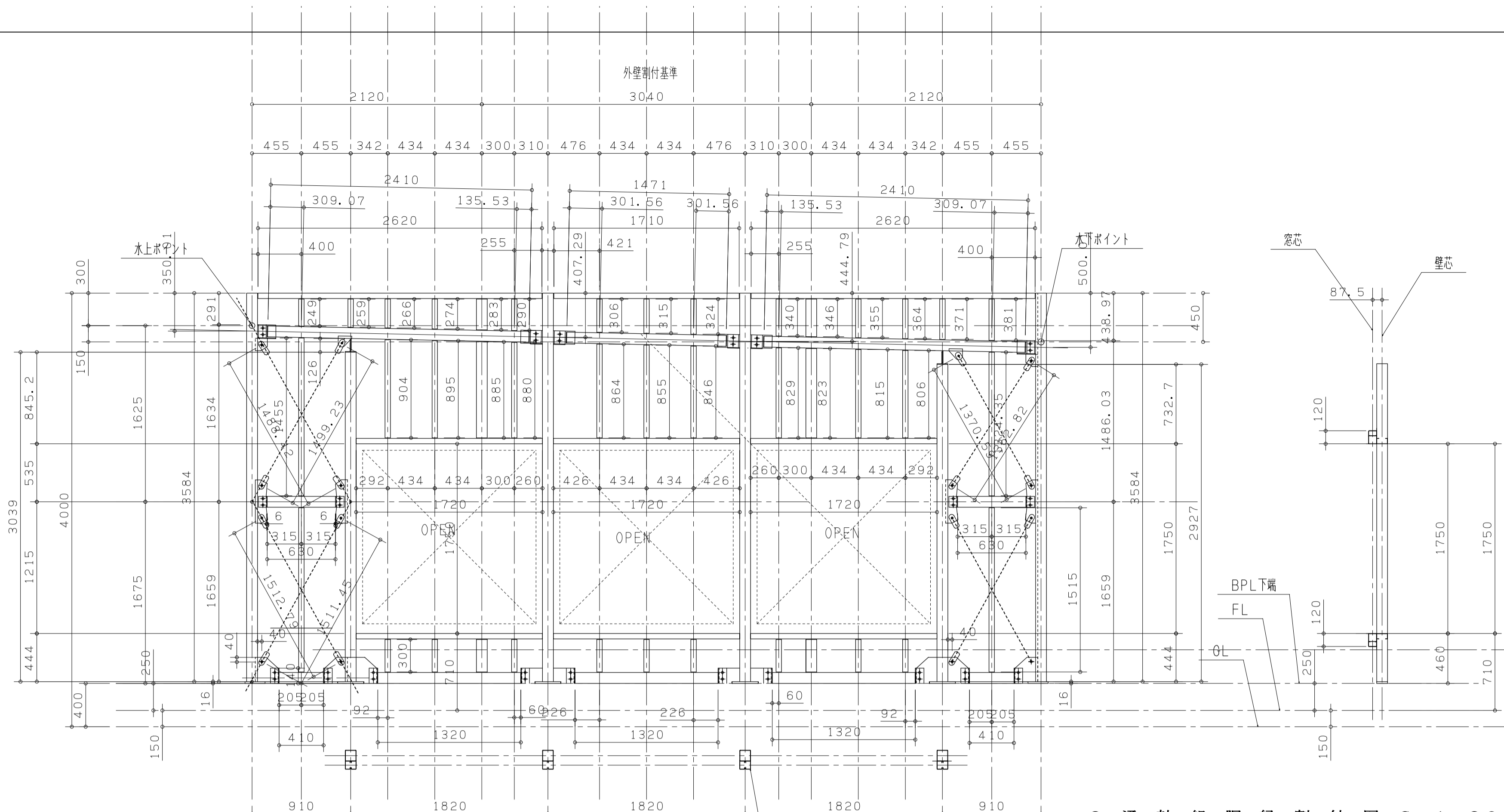
8 通軸組胴縁割付図 S=1:30
