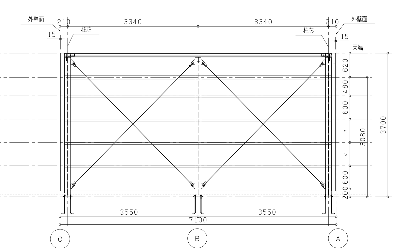
1.4 通軸組図 S=1:50
