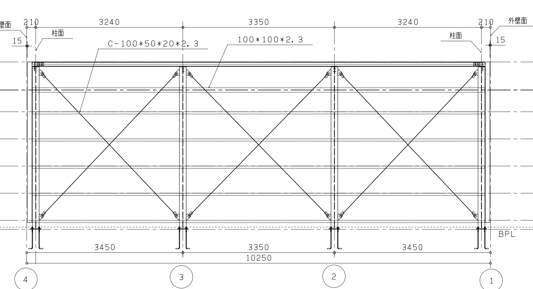
C 通軸組図 S=1:50
