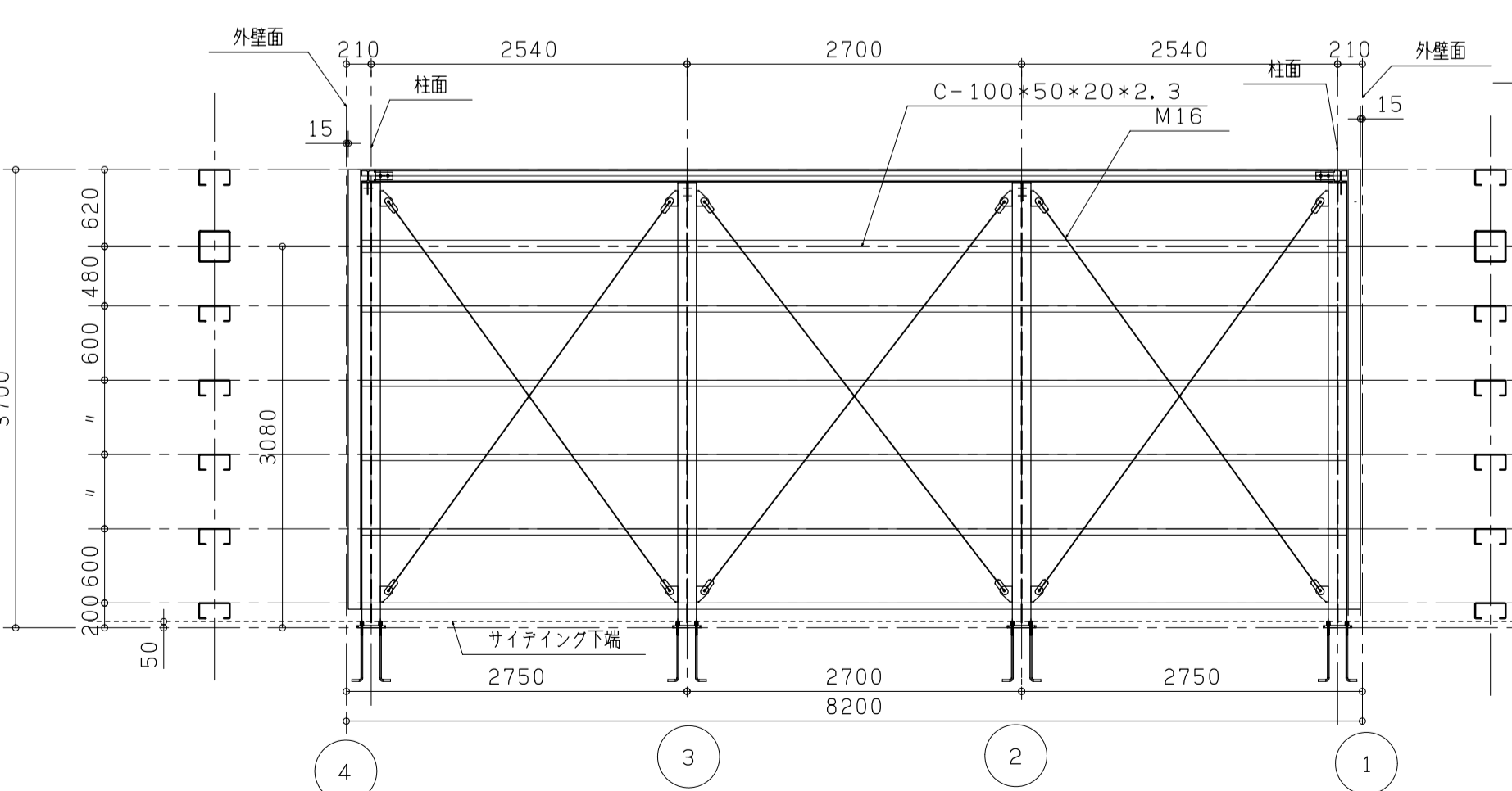
C 通軸組図 S=1:50
