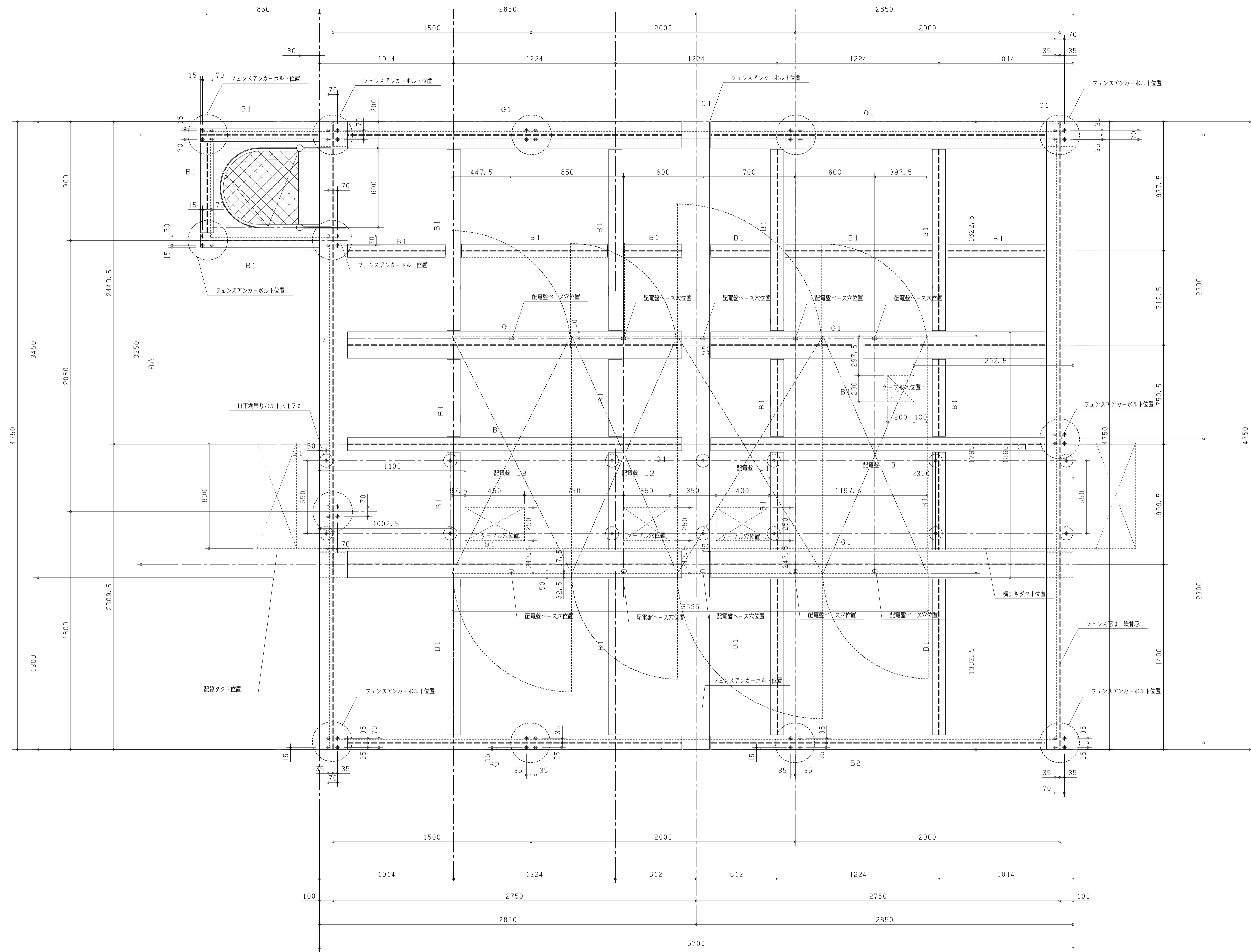
屋根アンカー位置図 S=1:15
