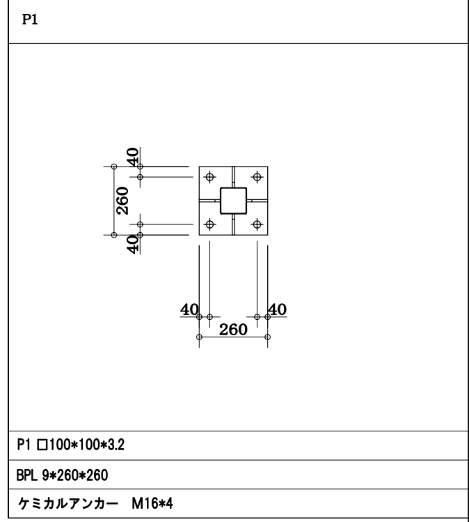
P1 □100*100*3.2 BPL 9*260*260 ケミカルアンカー M16*4
