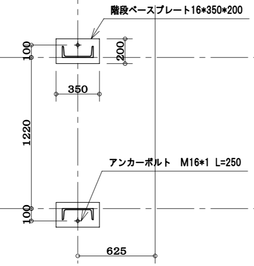
A~A断面図 S=1:30
