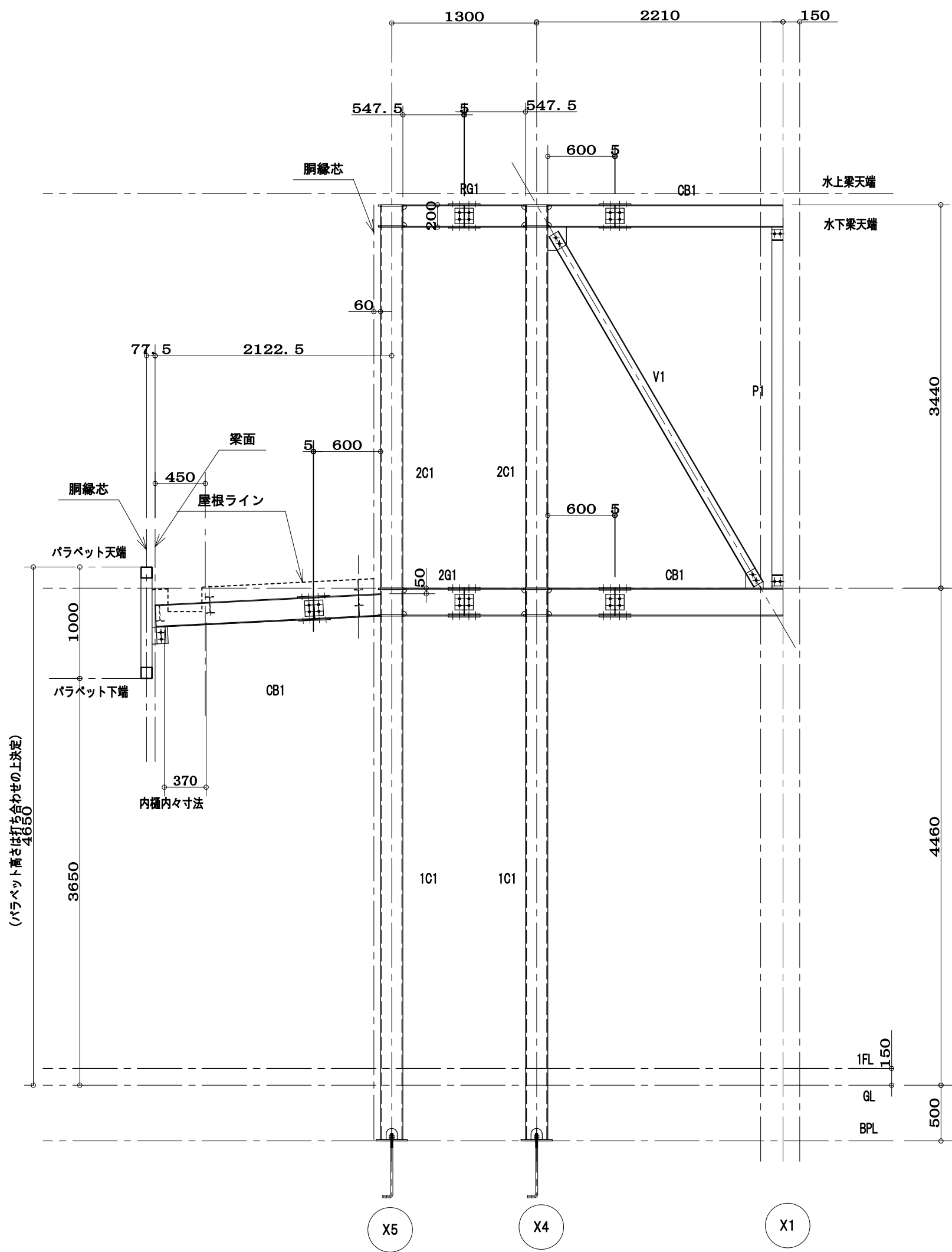
Y5 通軸組図 S=1:40
