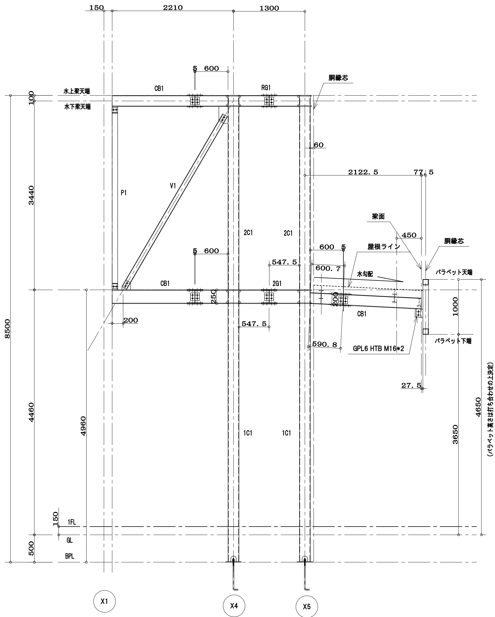
Y6 通軸組図 S=1:40
